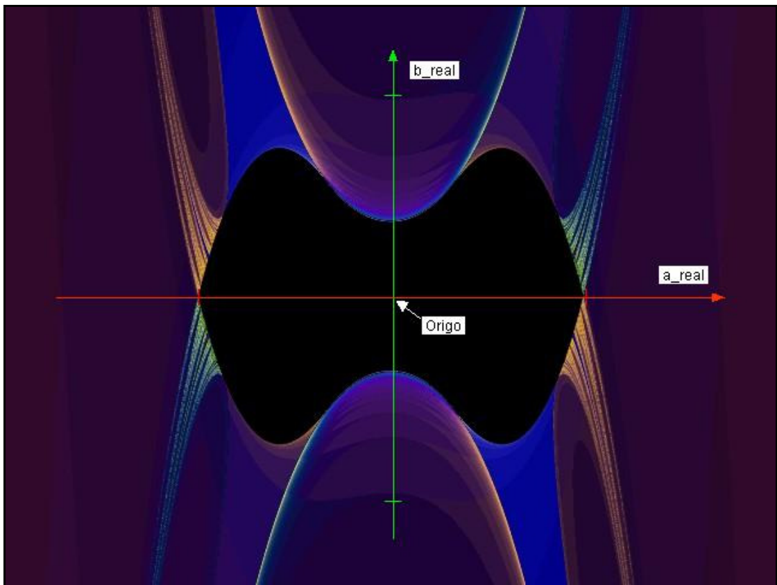
Fig 2. a_{\text{real}}, b_{\text{real}} .
