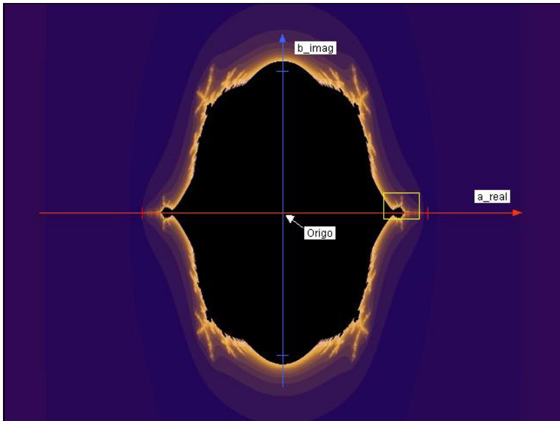
Fig 3. a_{\text{real}}, b_{\text{imag}} .
